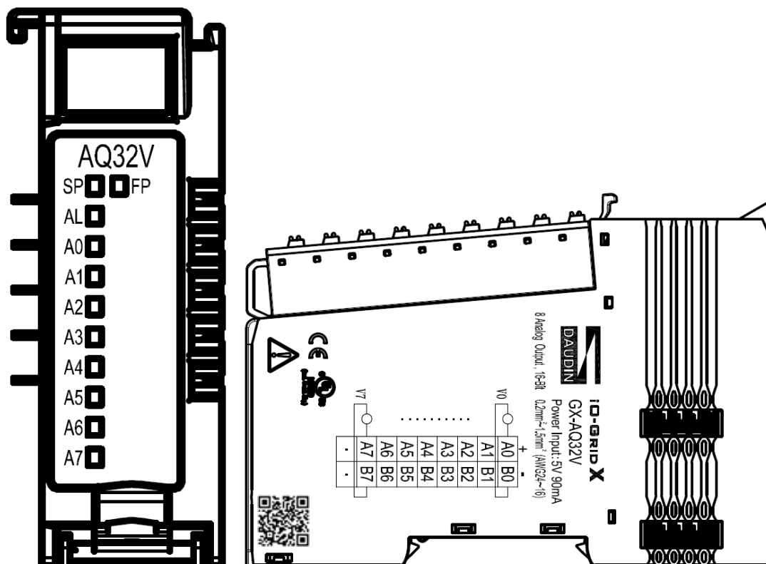
圖 4.31 GX-AQ32V 圖面
