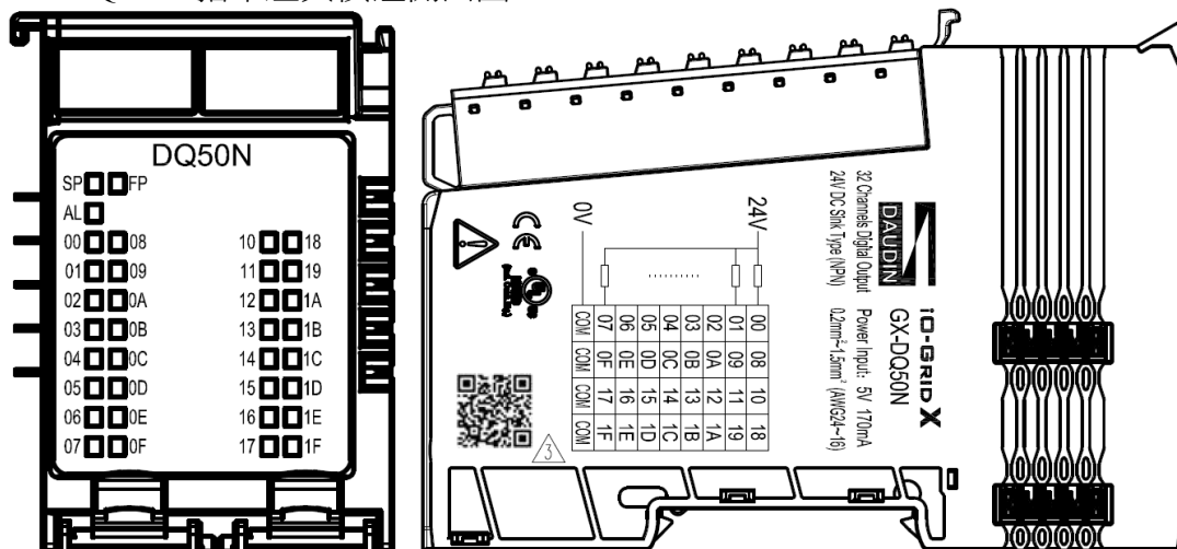
圖 4.13 GX-DQ50N 圖面
