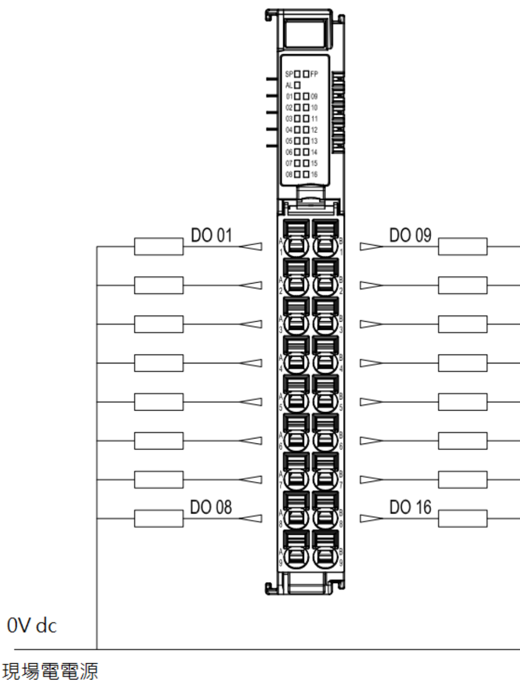
圖 8.9 GX-DQ40P 接線
