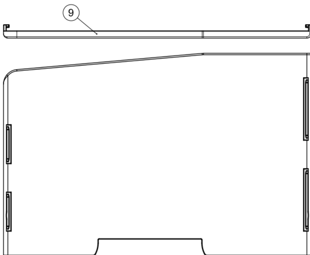
圖 4.1 側面蓋板圖
