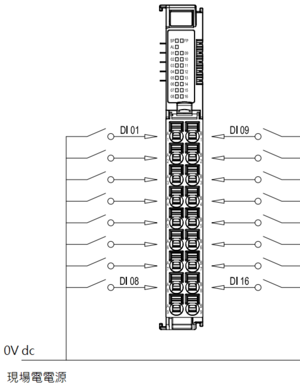
圖 8.2 GX-DI40N 接線圖
