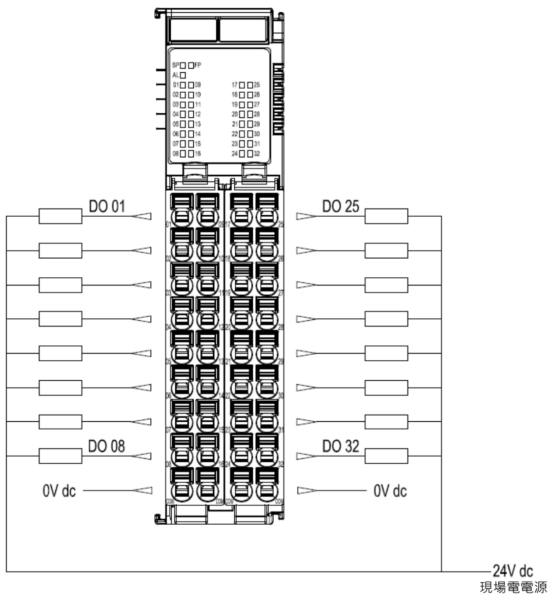
圖 8.10 GX-DQ50N 接線
