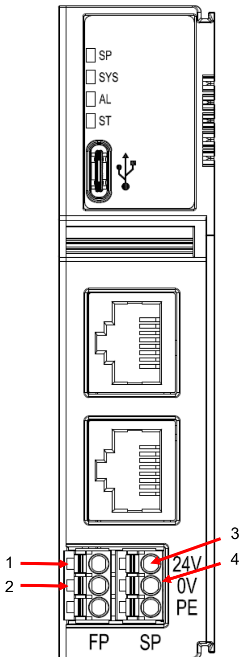
圖 3.2：電源
