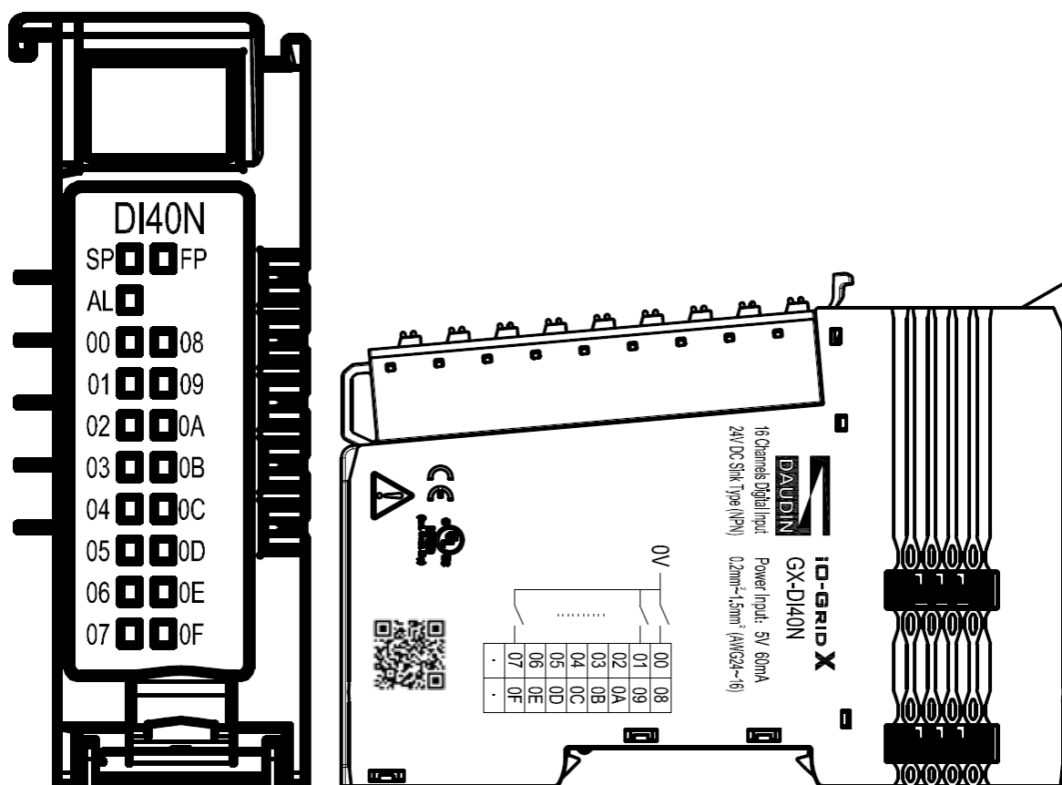
圖 4.4 GX-DI40N 圖面
