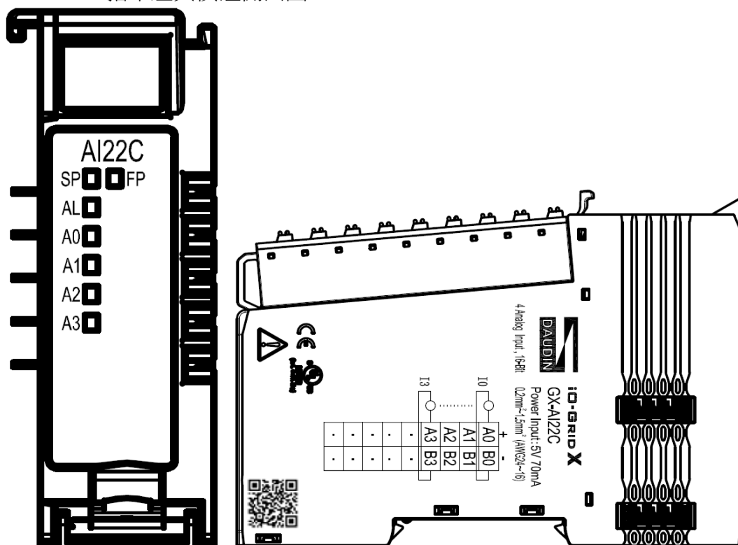
圖 4.20 GX-AI22C 圖面
