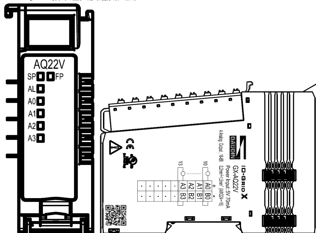
圖 4.27 GX-AQ22V 圖面
