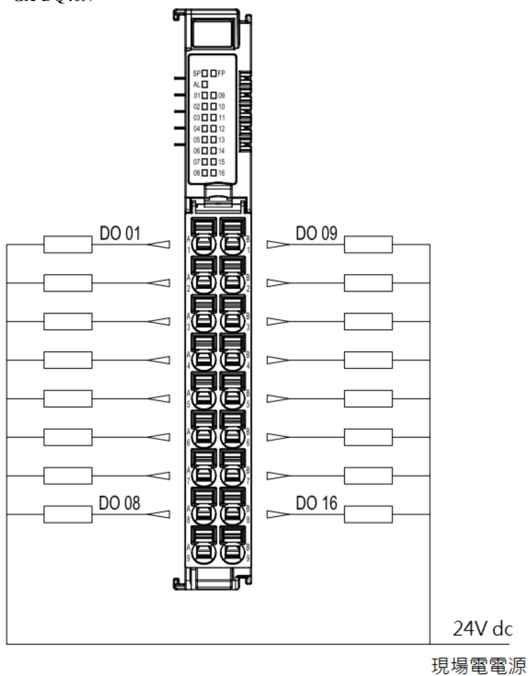
圖 8.8 GX-DQ40N 接線圖
