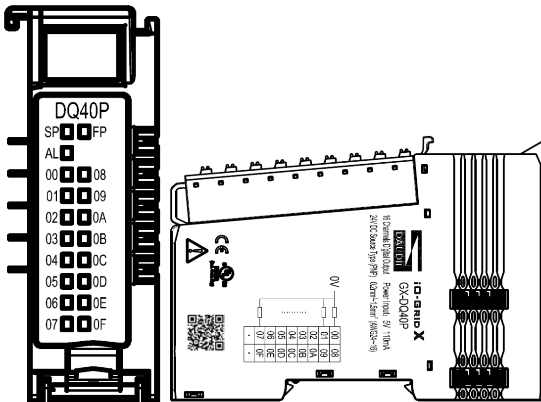
圖 4.12 GX-DQ40P 圖面
