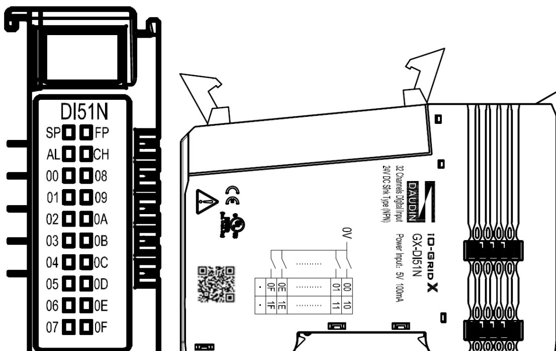
圖 4.9 GX-DI51N 圖面
